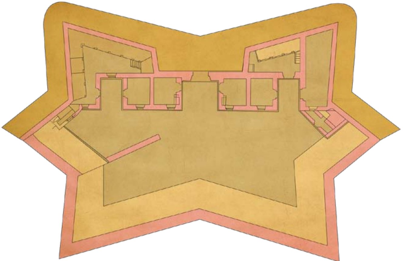
Plano de la batería de Doniños. Construcción antigua redibujada
